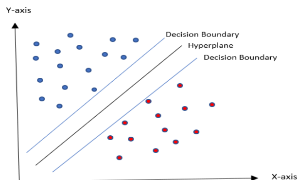
Fig. 3. SVM hyperplane
